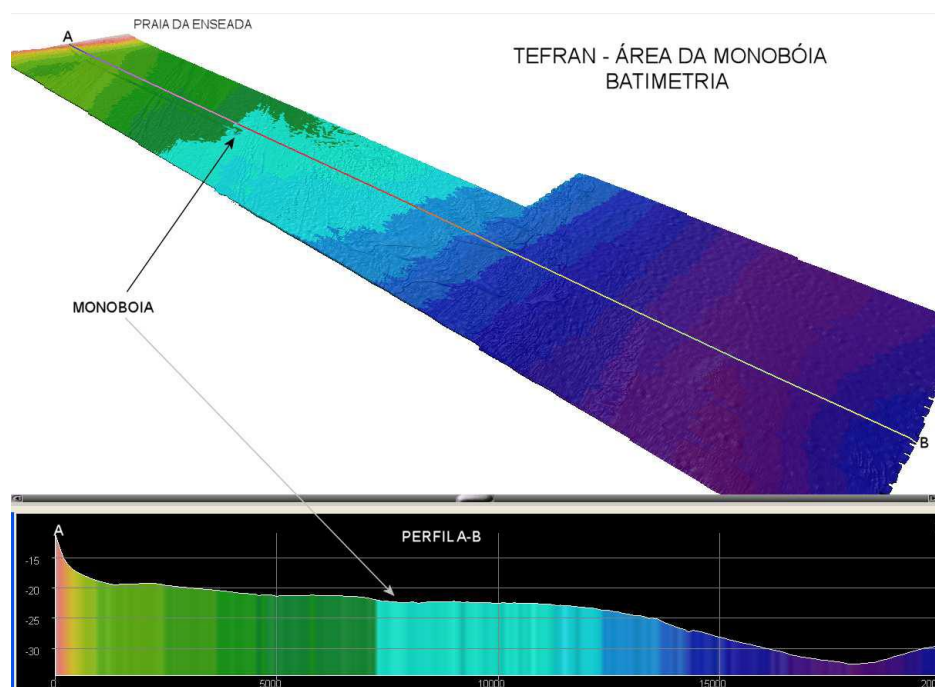
Figura 2 – Perfil batimétrico ao longo da área levantada
