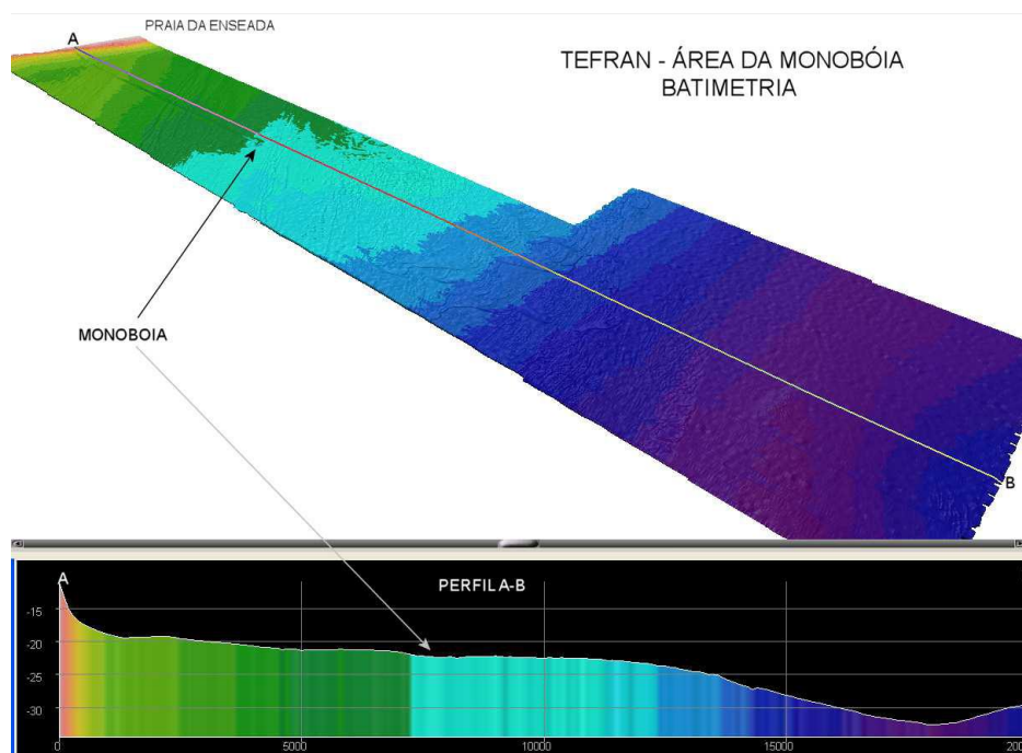
Figura 2 – Perfil batimétrico ao longo da área levantada
