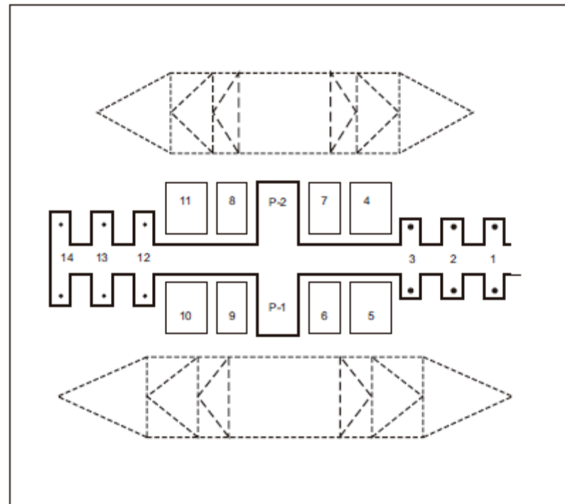
Figura 4 Esquema dos dólfinos do píer sul apresentado no Port Information.
