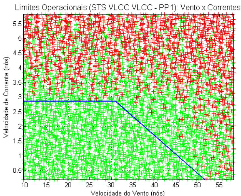
Figura 10 Limites operacionais para STS entre VLCCs no PP1 incluindo a restrição de capacidade dos gatos de desengate rápidos situado na plataforma de acostagem 9 (Figura 4)
