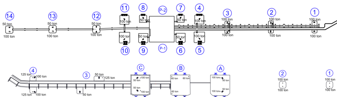
Figura 1 Planimetria do arranjo geral atual do Píer Sul (acima) e Pier Norte (abaixo).
