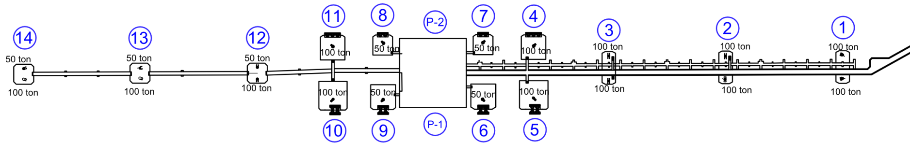
Figura 3 Planimetria do arranjo geral atual do Píer Sul.
