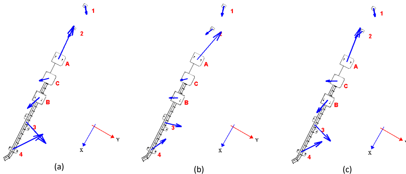
Figura 8 Exemplo gráfico de casos que produziram elevadas cargas longitudinais no Píer Norte. (a) 2 Suezmax atracados ao PP3 e 1 Panamax atracado ao PP4; (b) 2 Aframax no PP3 e 2 Panamax no PP4; (c) 2 Suezmax carregados no PP3 e 2 Panamax no PP4
