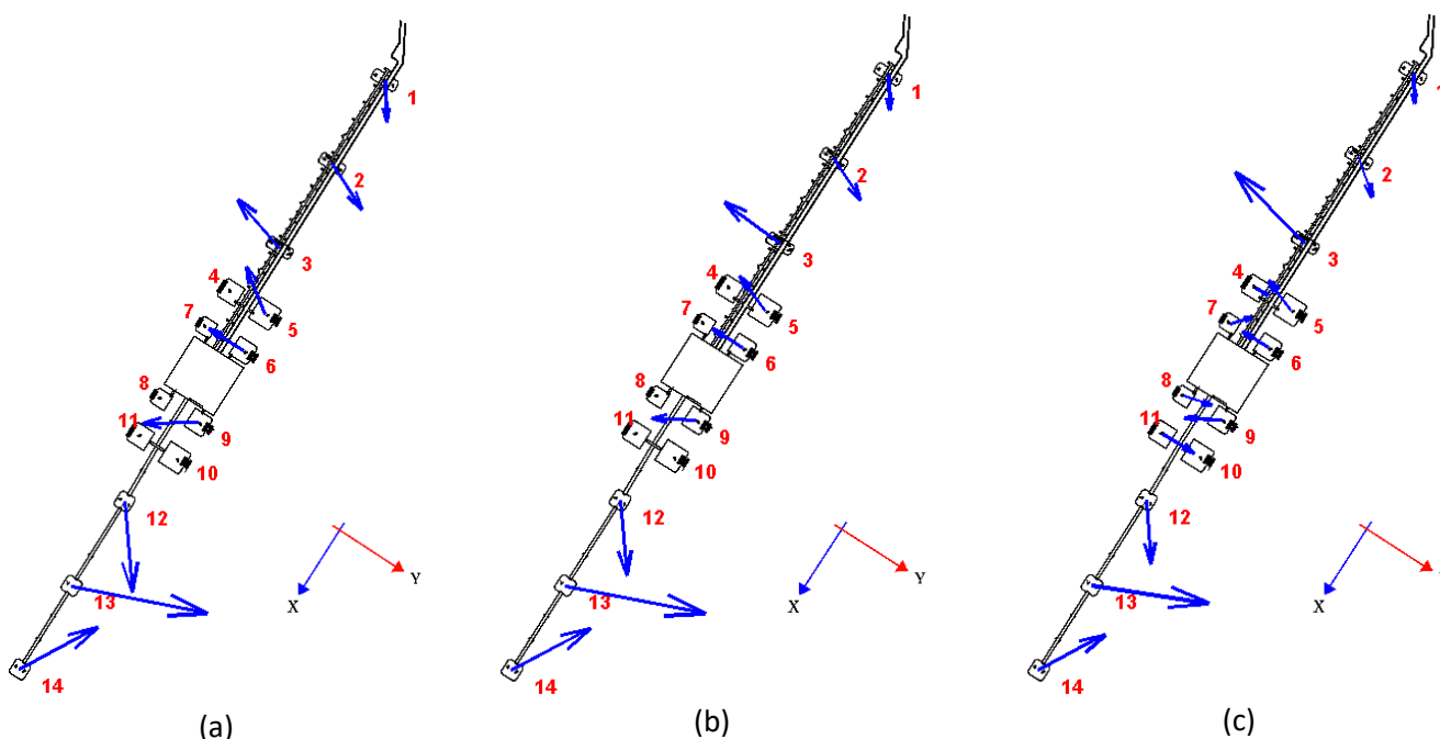
Figura 7 Exemplo gráfico de casos que produziram elevadas cargas transversais no Píer Sul. (a) 2 VLCCs atracados ao PP1; (b) 2 VLCCs no PP1 e 2 Suezmax no PP3; (c) 2 VLCCs Carregados no PP1 e 2 Suezmax no PP2
