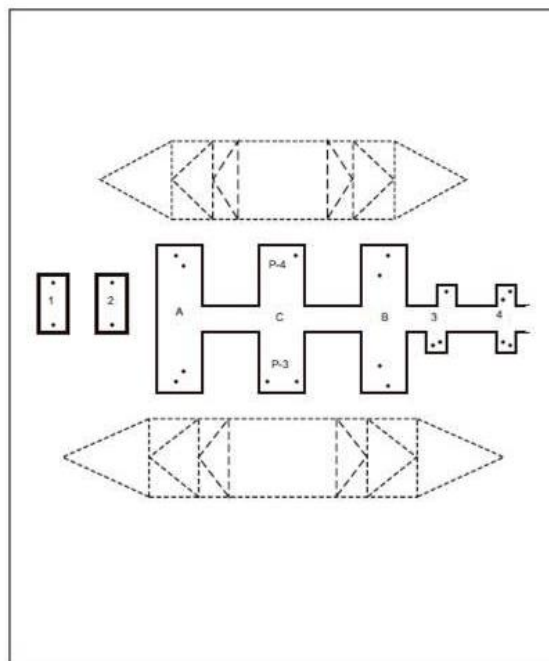
Figura 6 Esquema dos dólfins do píer norte apresentado no Port Information
