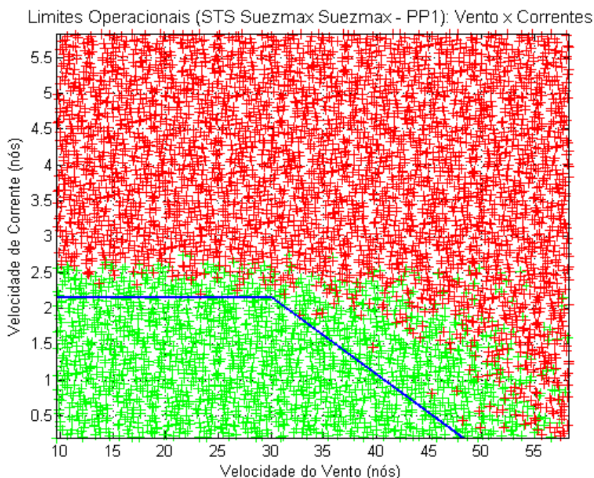
Figura 11 Limites operacionais para STS entre dois Suezmax no PP1 incluindo a restrição de capacidade dos gatos de desengate rápidos situado na plataforma de acostagem 9 (Figura 4)
