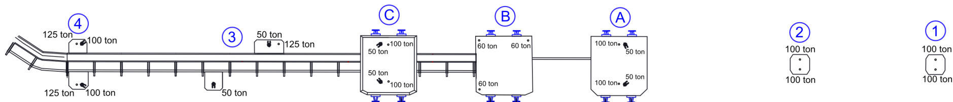
Figura 5: Planimetria do arranjo geral atual do Píer Norte.
